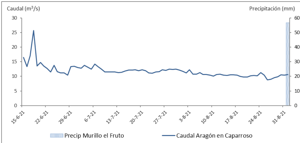
Gráfico 2. Caudales medios diarios en m 3 /s en la estación de aforo de Aragón en Caparroso (CHE) y precipitación acumulada diaria en l/m 2 en la estación meteorológica de Murillo el Fruto entre el 15-06-2021 y el 01-09-2021. Fuente de datos: Web del Agua de Navarra, Mete Navarra y CHE. Elaboración propia. Los datos son provisionales y están sujetos a revisión.
