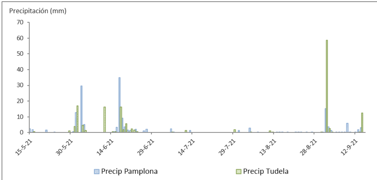
Gráfico 1. Precipitación acumulada diaria en l/m 2 en la estación meteorológica de Pamplona y en la de Tudela Montes del Cierzo entre el 15-05-2021 y el 15-09-2021. Fuente de datos: Mete Navarra. Elaboración propia. Los datos son provisionales y están sujetos a revisión.
