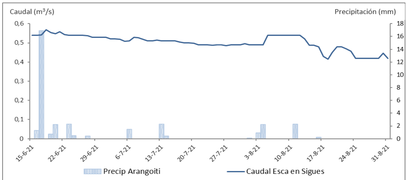
Gráfico 3. Caudales medios diarios en m 3 /s en la estación de aforo de Esca en Sigüés (CHE) y precipitación acumulada diaria en l/m 2 en la estación meteorológica de Arangoiti entre el 15-06-2021 y el 31-08-2021. Fuente de datos: Web del Agua de Navarra, MeteoNavarra y CHE. Elaboración propia. Los datos son provisionales y están sujetos a revisión.
